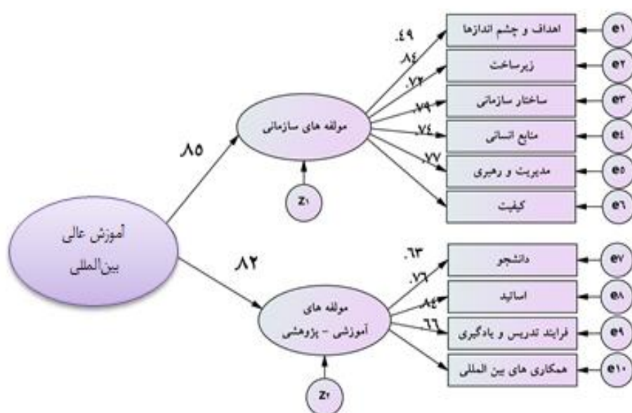
شکل ۱. مدل عاملی مرتبه دوم مفهوم آموزش عالی بین‌المللی
